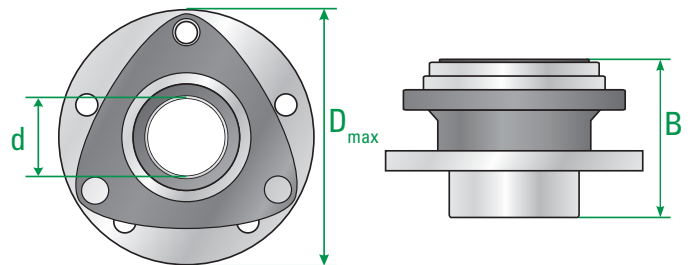
Roulement de roue Génération 3
