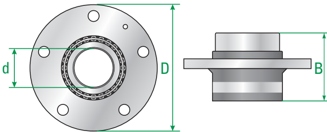
Radlager Generation 2.1
