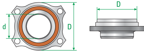
Cuscinetto Generazione 2D
