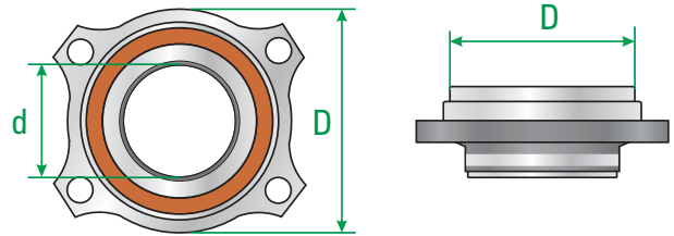
Roulement de roue Génération 2D
