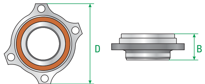
Rodamiento Generación 3
