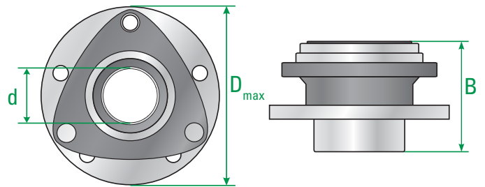
Radlager Generation 3
