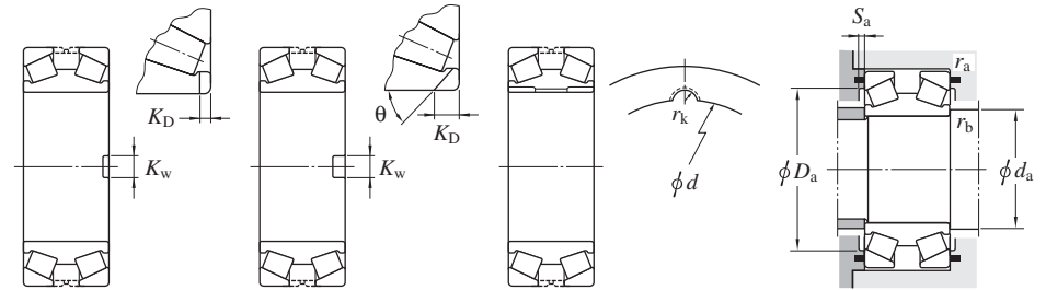
Face key way : A Face key way : B Bore key way
